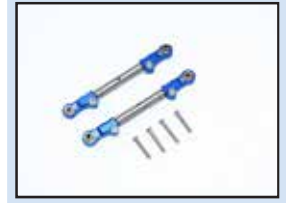
Art.Nr.: GPMTXMS162SB Alum. Kugelpfannen mit Edelstahl Spurstangen Lenkung blau
